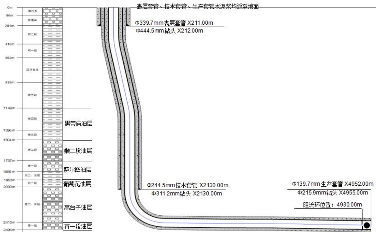
图 3.2-1 井身结构示意图
