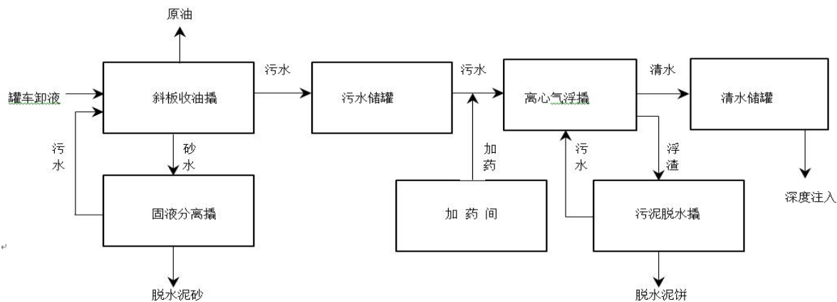
图3.6-1 压裂返排液处理主要工艺流程
