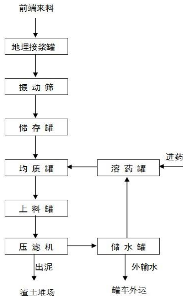
图 3.6-2 采油九厂 15 万 m 3 /a 钻井废弃泥浆无害化处理站工艺流程图
