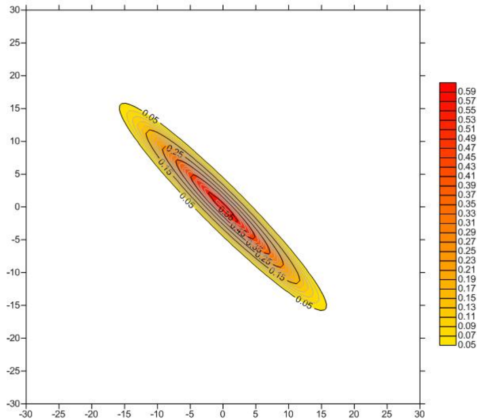
图 5.3-2 泥浆槽泄漏 100d 石油类预测范围图
