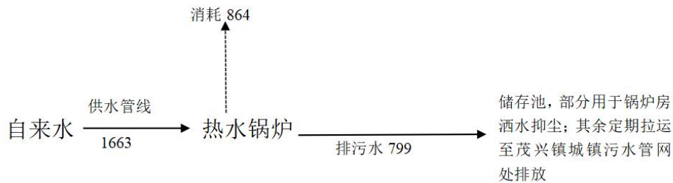
图 2-1 建设项目水平衡图（单位:t/a）
